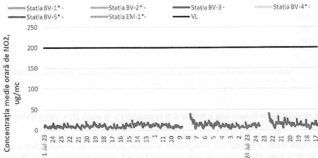
Figura 1.1.2.2.1. Evoluția mediilor orare de \text{NO}_2 în luna iulie
