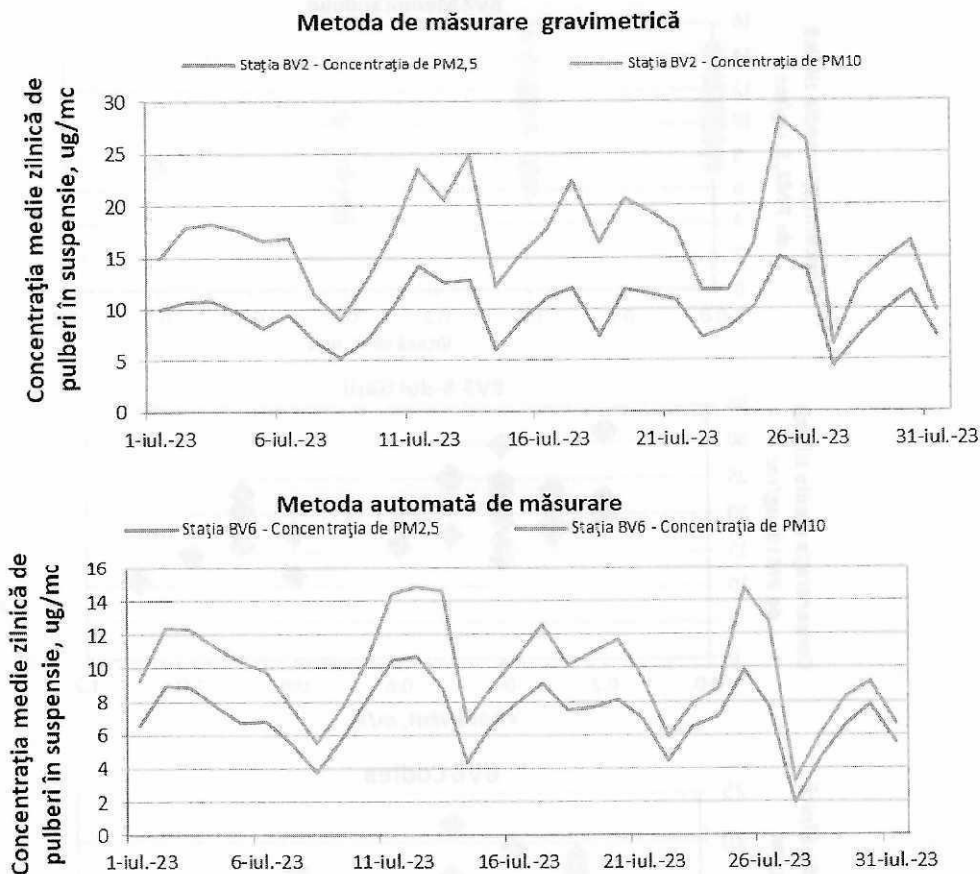
Figura 1.1.2.4.4 Evoluția mediilor zilnice de PM 2,5 și PM10 în luna iulie
