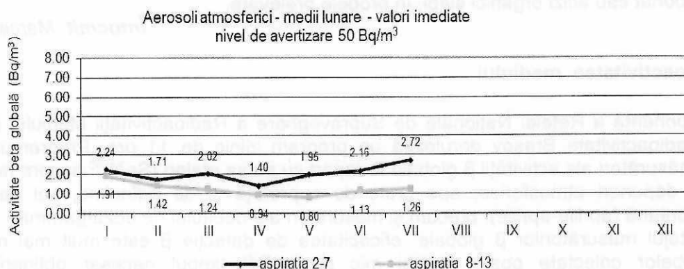
Fig. 1.2.1. Activitatea beta globală pentru aerosoli atmosferici
