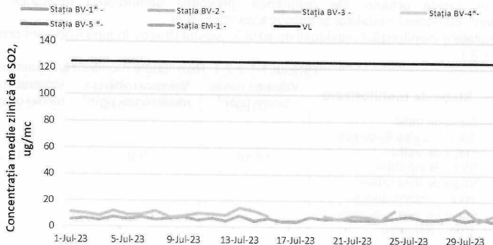
Figura 1.1.2.1.1. Evoluția mediilor zilnice de \text{SO}_2 în luna iulie
