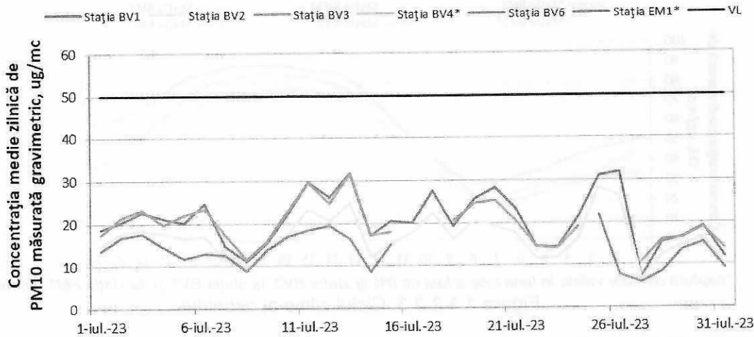
Figura 1.1.2.4.1. Evoluția mediilor zilnice de PM 10 (gravimetric) în luna iulie
