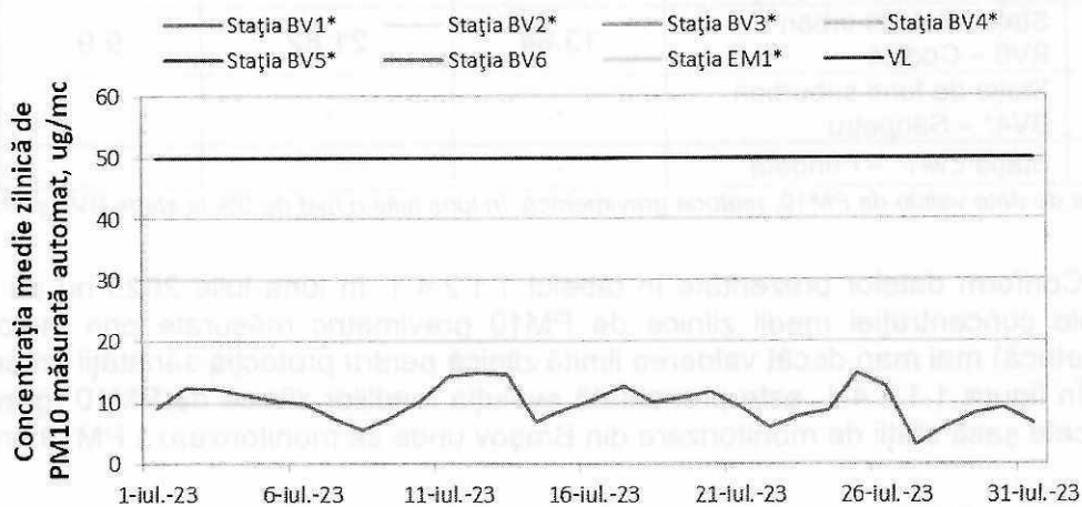
Figura 1.1.2.4.3. Evoluția mediilor zilnice de PM 10, metoda automată, în luna iulie
